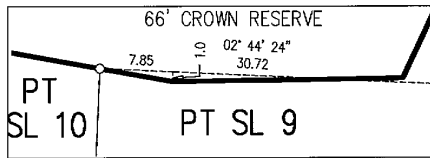
DETAIL B SCALE: 1:500
